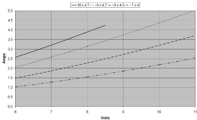
C 2212-0840 Strom über Spannung mit versch. Luftschrauben
