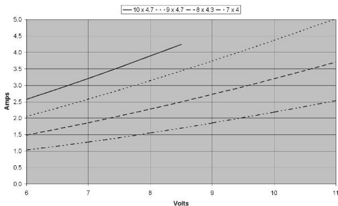
C 2212-0840 courant/tension avec différentes hélices
