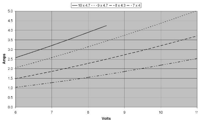
C 2212-0840 Corrente e tensione con eliche diverse
