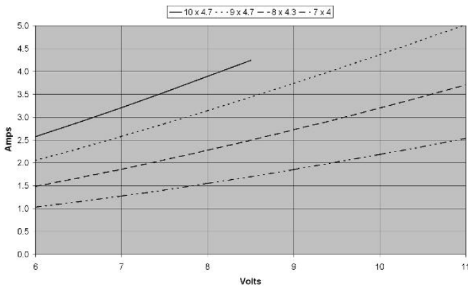
C 2212-0840 Consumo y voltaje con distintas hélices
