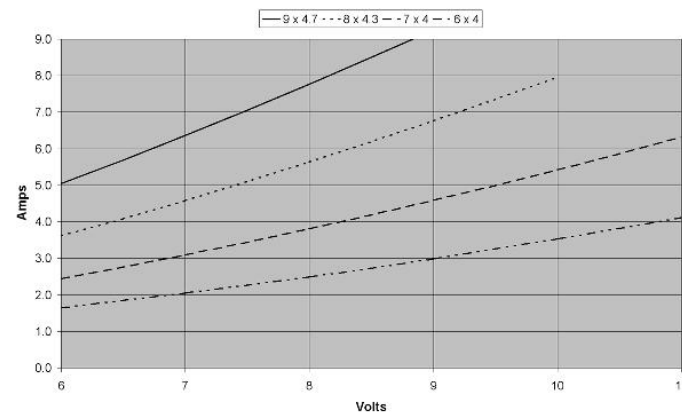
C 2212-1180 Strom über Spannung mit versch. Luftschrauben
