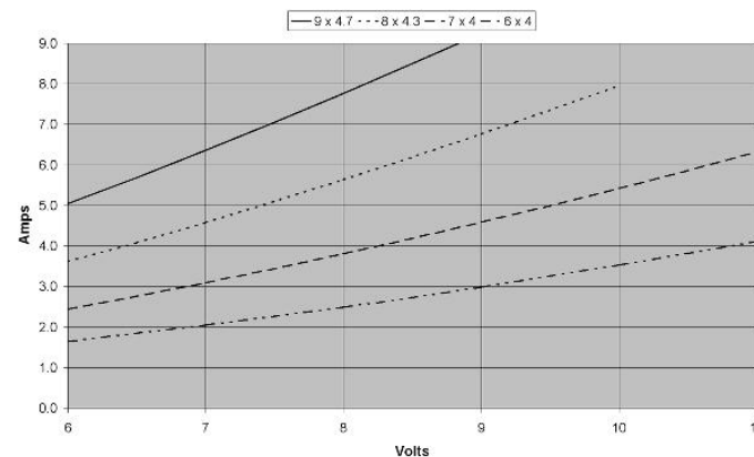
C 2212-1180 Corrente e tensione con eliche diverse
