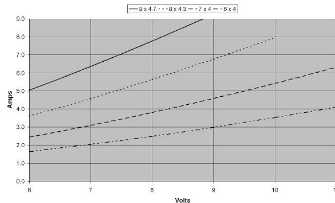
C 2212-1180 Consumo y voltaje con distintas hélices
