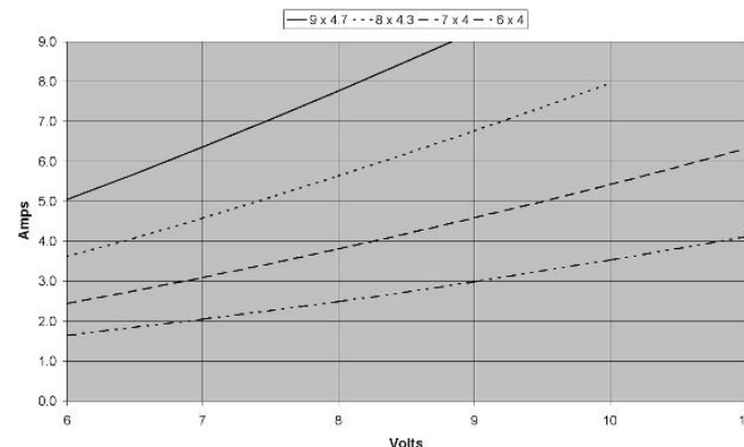
C 2212-1180 courant/tension avec différentes hélices
