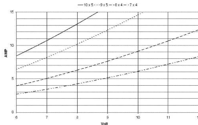
C 2808-1160 Consumo y voltaje con distintas hélices
