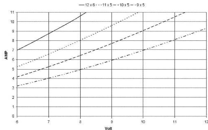
C 2808-0860 Consumo y voltaje con distintas hélices
