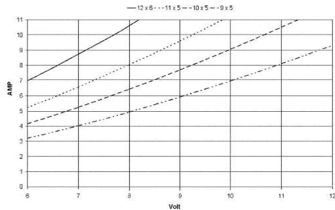
C 2808-0860 Strom über Spannung mit versch. Luftschrauben
