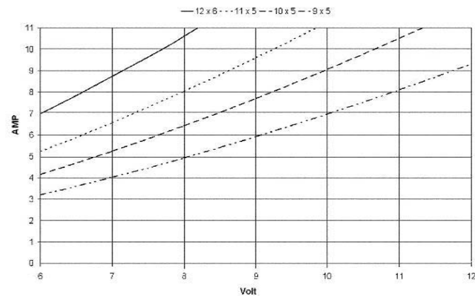
C 2808-0860 courant/tension avec différentes hélices
