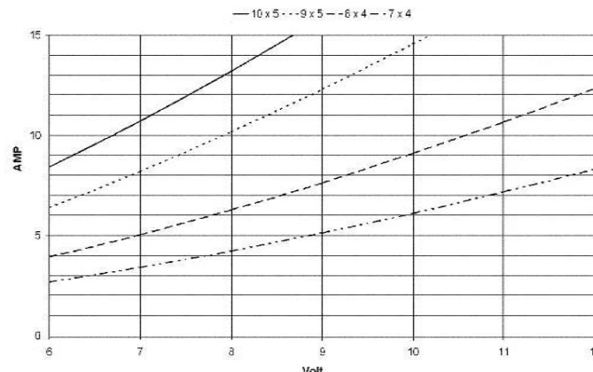
C 2808-1160 Strom über Spannung mit versch. Luftschrauben
