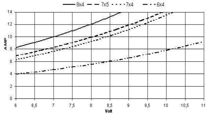
C 2808-1550 Strom über Spannung mit versch. Luftschrauben
