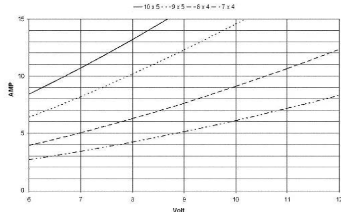
C 2808-1160 courant/tension avec différentes hélices
