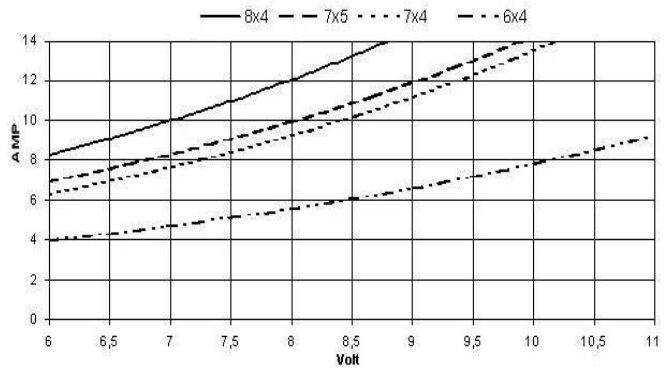
C 2808-1550 Consumo y voltaje con distintas hélices
