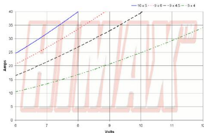
C 3510-1540 Corrente e tensione con eliche diverse
