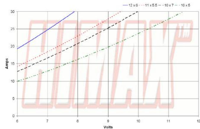
C 3510-1100 Consumo y voltaje con distintas hélices
