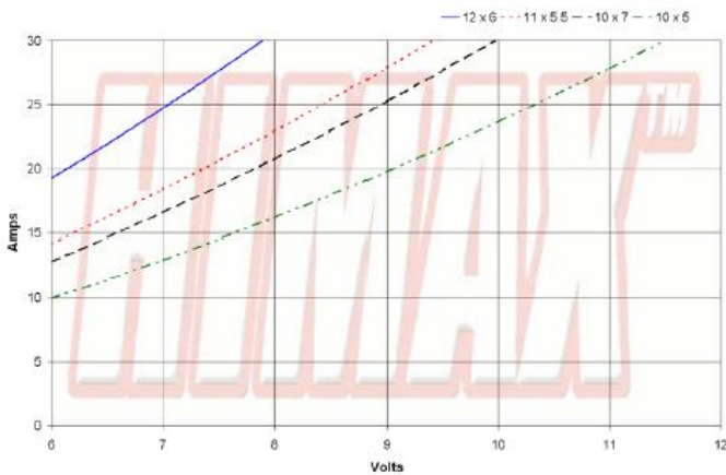
C 3510-1100 Corrente e tensione con eliche diverse
