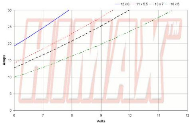
C 3510-1100 courant/tension avec différentes hélices
