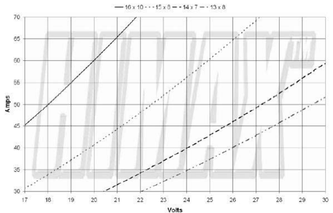
C 5030-0390 Consumo y voltaje con distintas hélices
