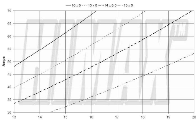
C 5018-0530 Strom über Spannung mit versch. Luftschrauben
