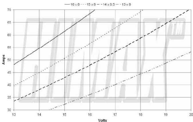
C 5018-0530 Consumo y voltaje con distintas hélices
