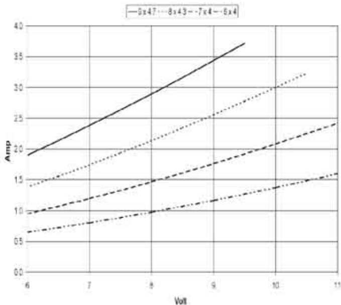
HC2208-0870 Strom und Spannung mit Luftschrauben
