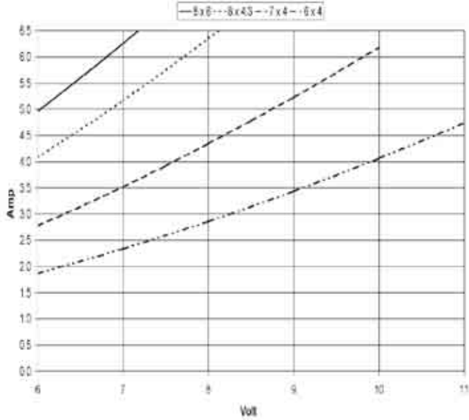
HC2208-1260 Strom und Spannung mit Luftschrauben
