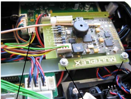
Connecteur "INT PPM"
