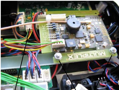
Steckplatz "INT PPM"
