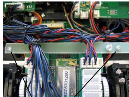
Schraubdome im Sender
