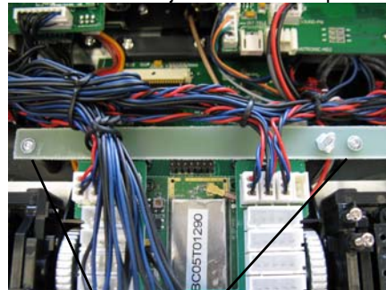
Pines en la emisora
