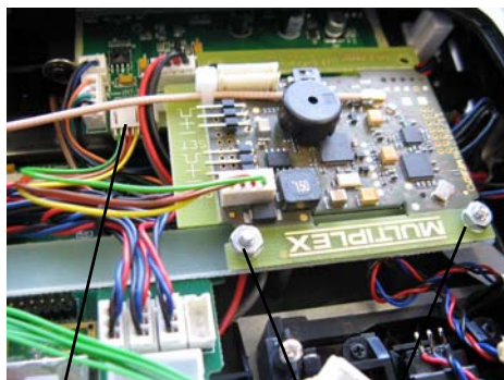
Slot "INT PPM" Rosetta e dado da M3
