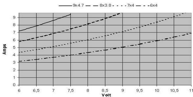
C 2805-1430 courant/tension avec différentes hélices
