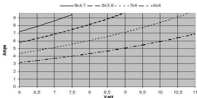
C 2805-1430 Consumo y voltaje con distintas hélices
