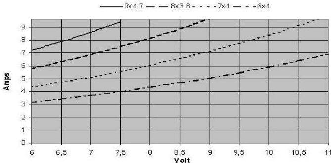
C 2805-1430 Strom über Spannung mit versch. Luftschrauben
