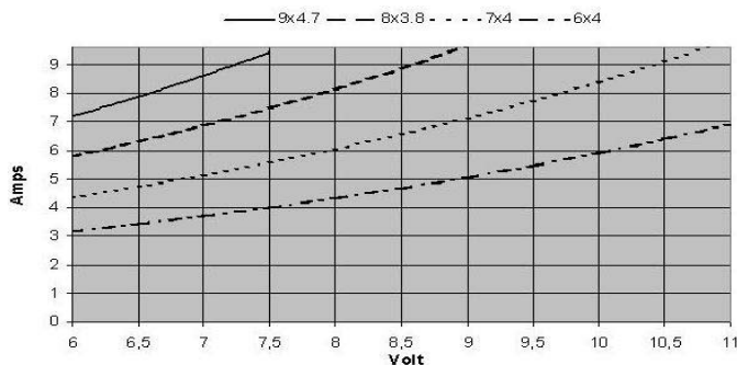
C 2805-1430 Corrente e tensione con eliche diverse
