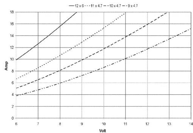
C 2816-0890 Corrente e tensione con eliche diverse
