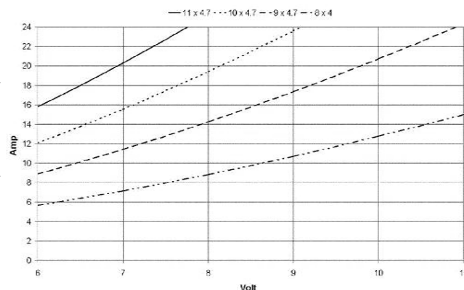
C 2816-1220 Corrente e tensione con eliche diverse
