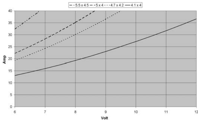
A 2825-3600 Corrente e tensione con eliche diverse
