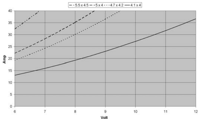
A 2825-3600 Strom über Spannung mit versch. Luftschrauben
