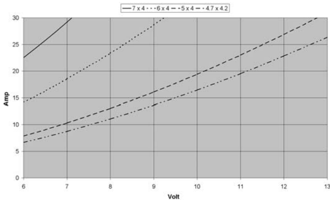
A 2825-2700 Corrente e tensione con eliche diverse
