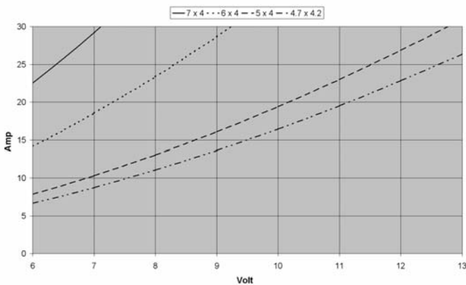
A 2825-2700 Consumo y voltaje con distintas hélices
