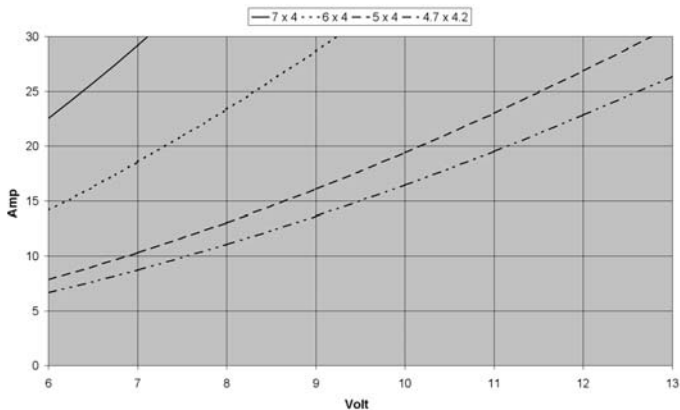
A 2825-2700 Strom über Spannung mit versch. Luftschrauben
