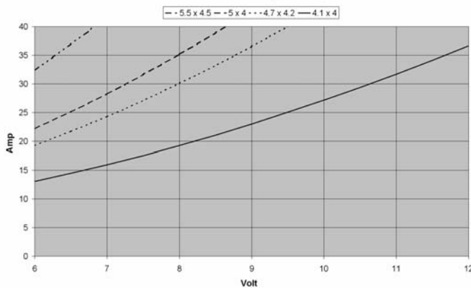
A 2825-3600 Consumo y voltaje con distintas hélices
