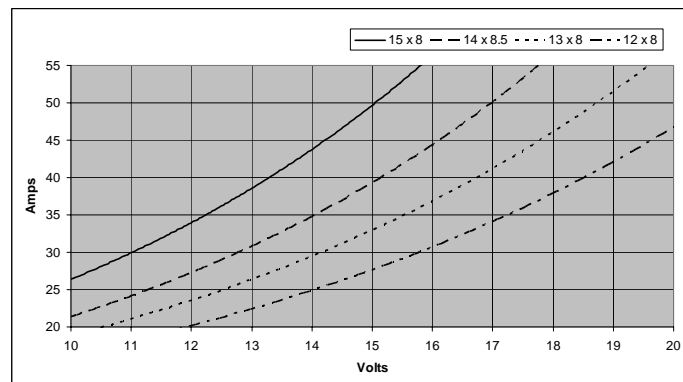
C 4220-0620 courant/tension avec différentes hélices
