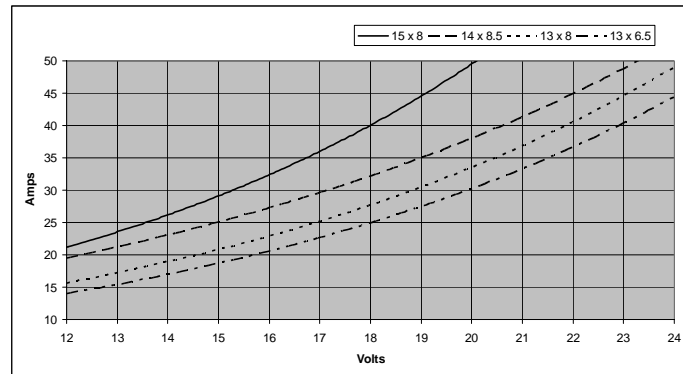
C 4220-0510 Strom über Spannung mit versch. Luftschrauben
