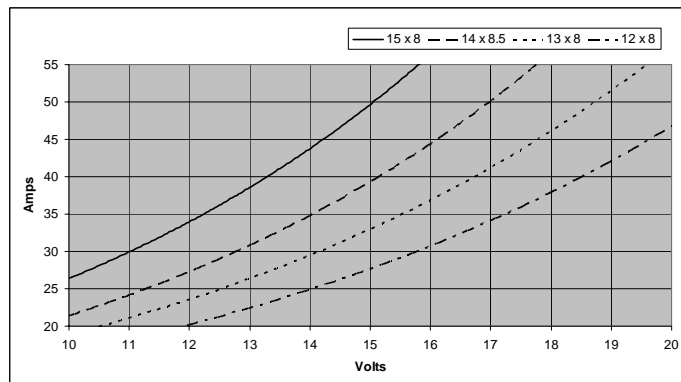
C 4220-0620 Consumo y voltaje con distintas hélices
