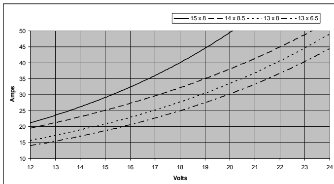
C 4220-0510 Corrente e tensione con eliche diverse
