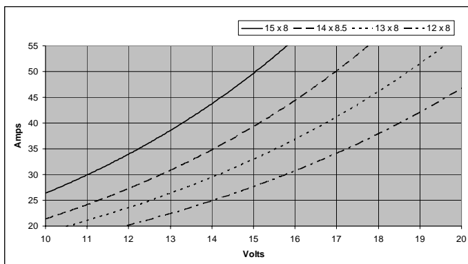
C 4220-0620 Corrente e tensione con eliche diverse
