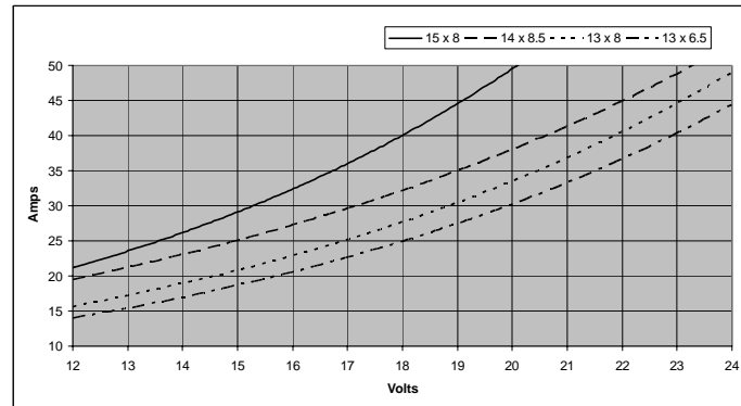
C 4220-0510 courant/tension avec différentes hélices
