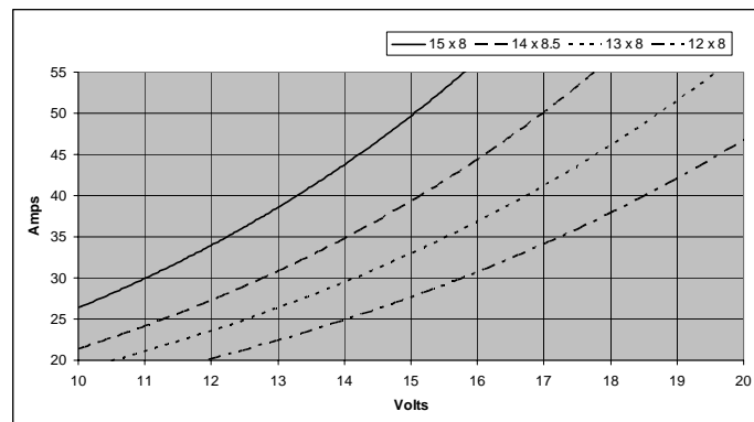
C 4220-0620 Strom über Spannung mit versch. Luftschrauben
