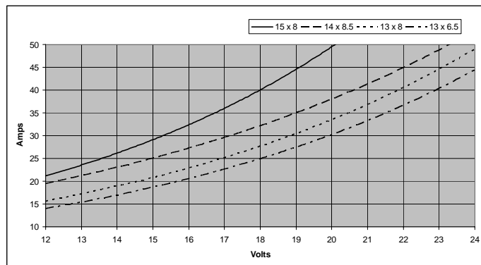
C 4220-0510 Consumo y voltaje con distintas hélices
